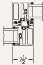
Interlockers
