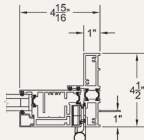
Hinge Side Jamb
