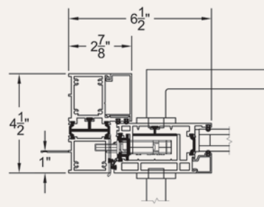
Lock Jamb
