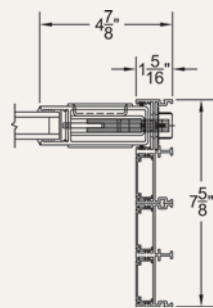
Lock Jamb
